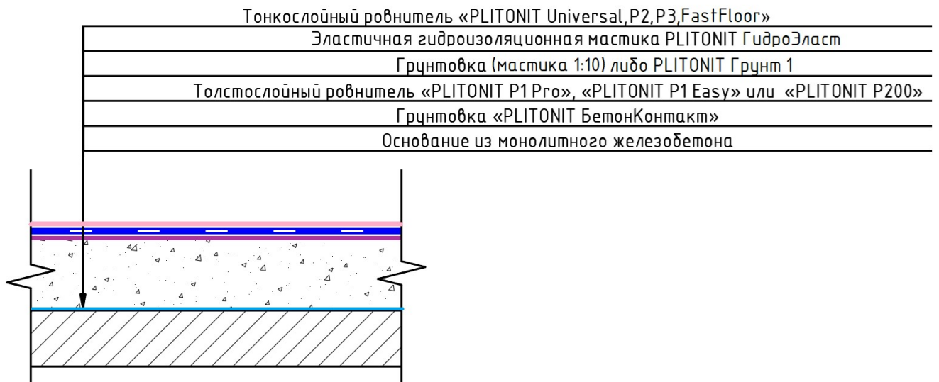
Сечение готового покрытия тонкослойного ровнителя.
