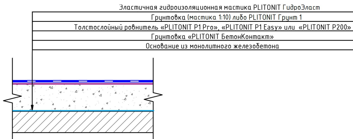
Сечение готового покрытия гидроизоляции.
